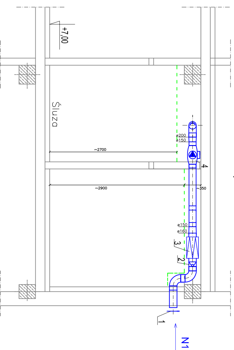
Przekrój 1-1
