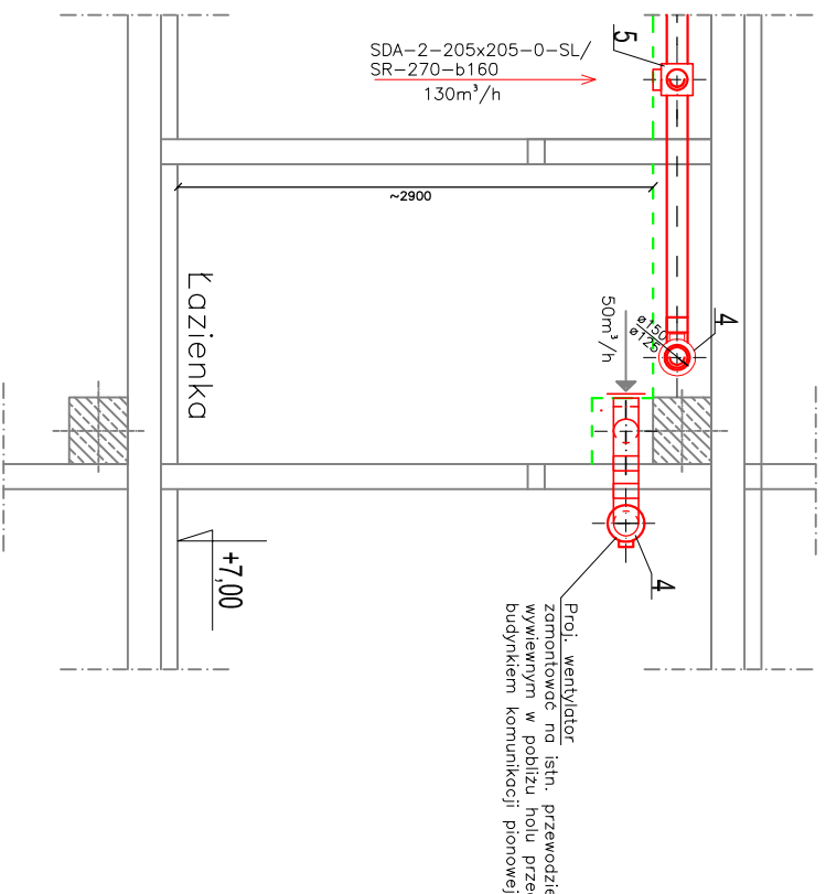
Przekrój 2-2
